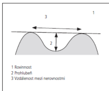
MĚŘENÍ ROVINNOSTI
