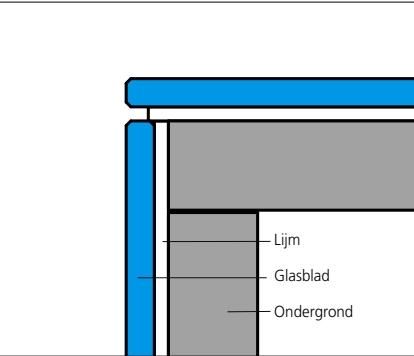
MEUBILAIR: DEUR EN HOEK
