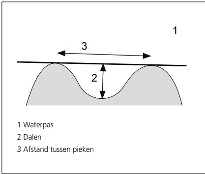
METING VAN VLAKHEID
