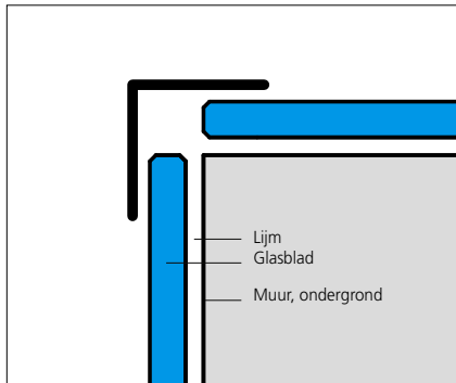
HOEKPROFIELEN: HOEKVORM
