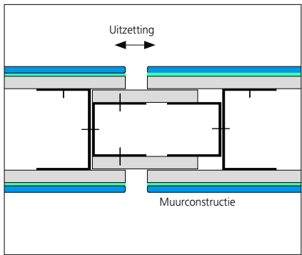
UITZETVOEG: MUUR
