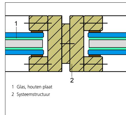
HOUTEN CONSTRUCTIE: HORIZONTALE DWARSDOORSNEDE
