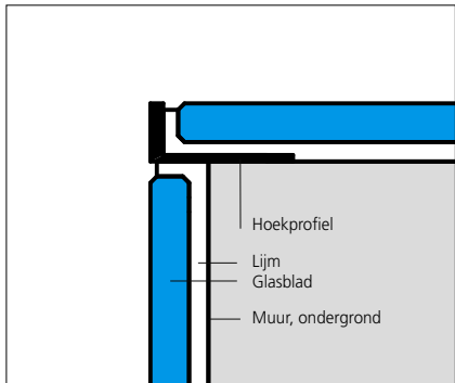
HOEKPROFIELEN: L-VORM
