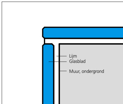
GLASHOEK: GLASVOEG
