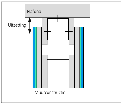
GLIJDENDE VOEG: PLAFOND
