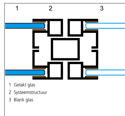
METALEN STRUCTUUR: HORIZONTALE DWARSDOORSNEDE
