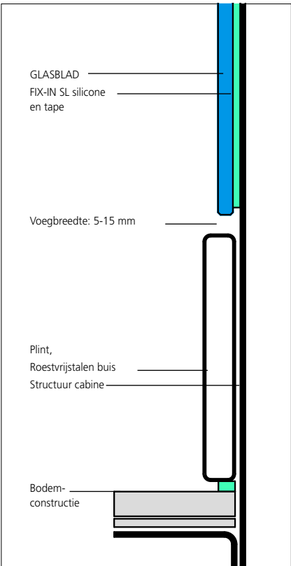
LIFTCABINE: VERTICALE DWARSDOORSNEDE MET PLINT
