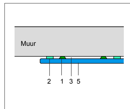
HORIZONTALE DOORSNEDE
