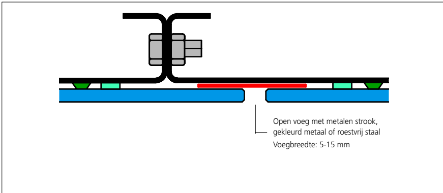
LIFTCABINE: HORIZONTALE DWARSDOORSNEDE MET GEKLEURDE VOEG
