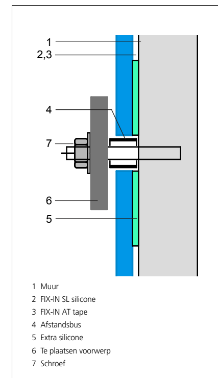
PLAATSING MET AFSTANDBUS
