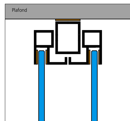
METALEN STRUCTUUR: VERTICALE DWARSDOORSNEDE
