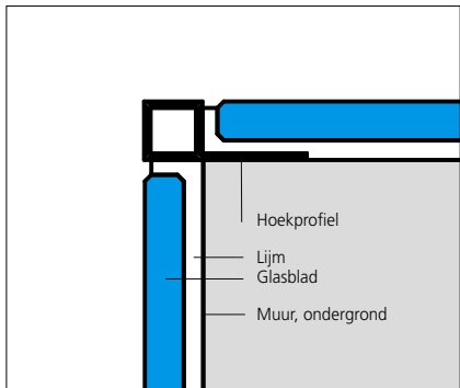
HOEKPROFIEL: VIERKANT
