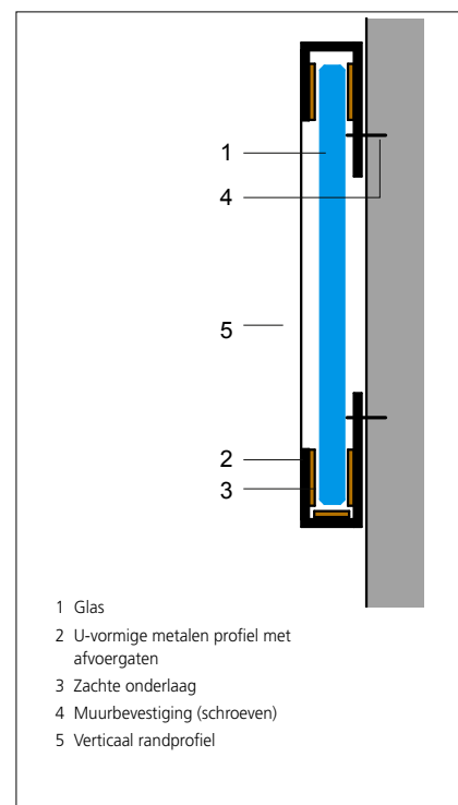
MECHANISCHE BEVESTIGING: MIROX
