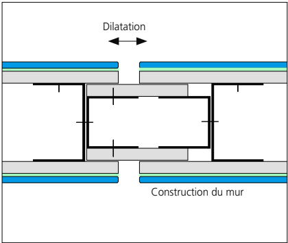
JOINT DE DILATATION : MUR
