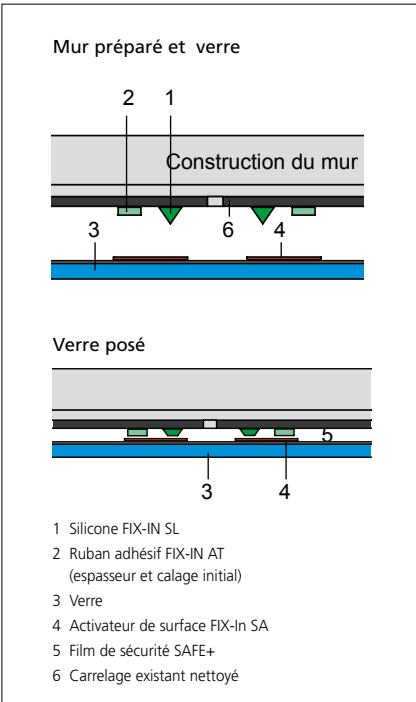
VERRE AVEC FILM DE SÉCURITÉ SAFE+
