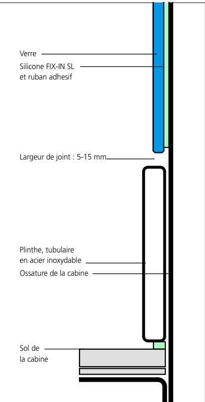
CABINE D'ASCENSEUR : COUPE VERTICALE AVEC PLINTHE
