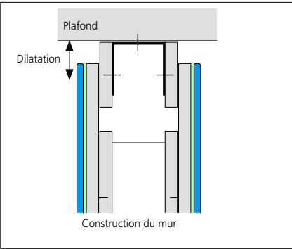
JOINT COULISSANT : PLAFOND
