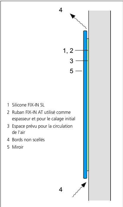
COUPE VERTICALE
