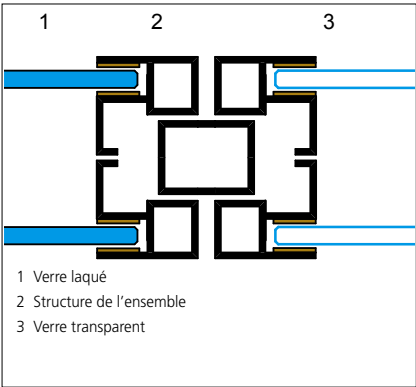
OSSATURE METALLIQUE : COUPE HORIZONTALE
