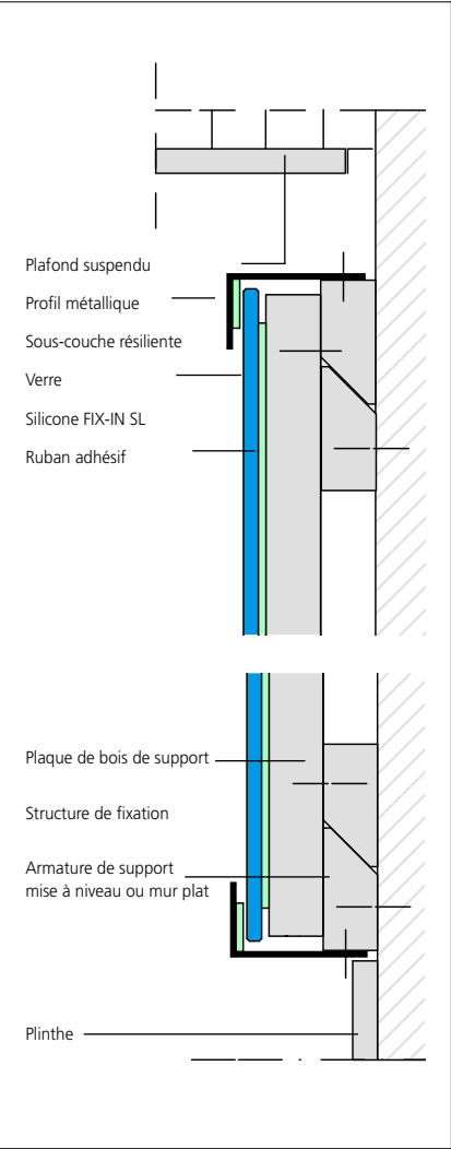
COUPE VERTICALE
