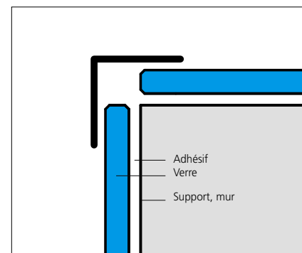
PROFILS D'ANGLE : FORME EN COIN
