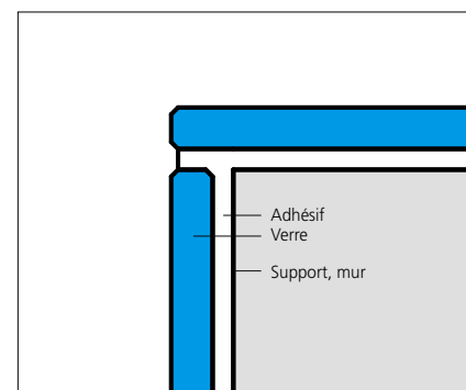
VERRE EN ANGLE JOINT
