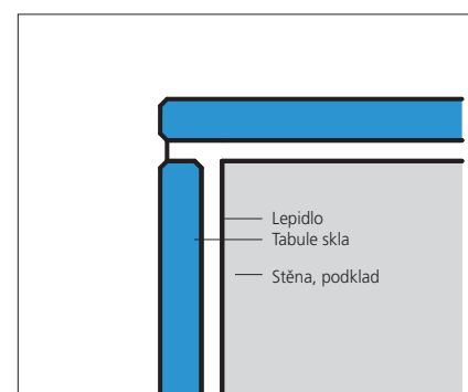
ROH TVOŘENÝ SKLY: SPÁRA MEZI SKLY
