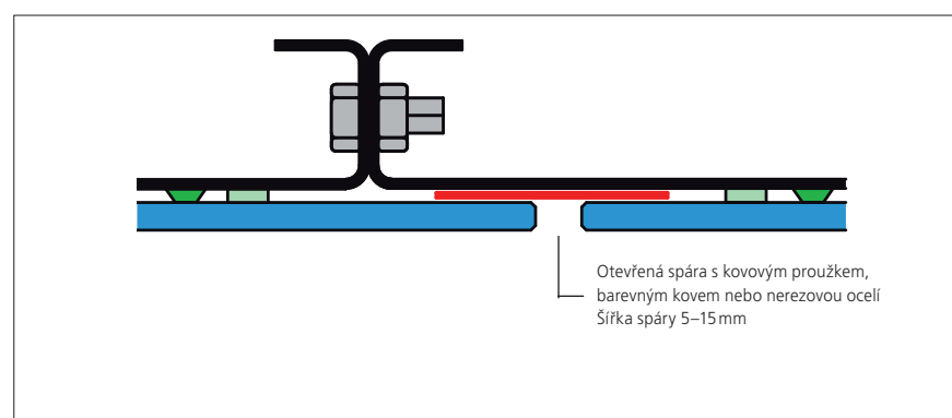
KABINA VÝTAHU: VODOROVNÝ ŘEZ S BAREVNOU SPÁROU
