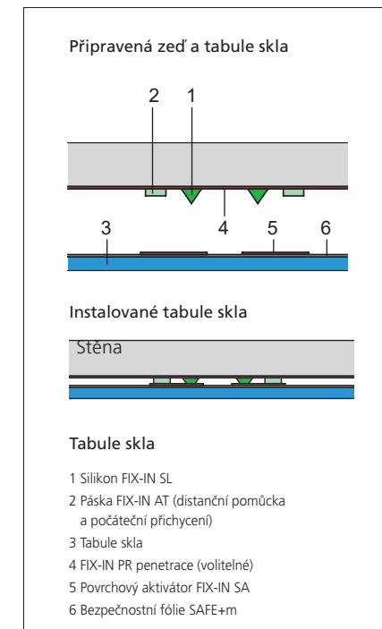
SKLO S BEZPEČNOSTNÍ FÓLIÍ SAFE+
