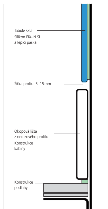
KABINA VÝTAHU: SVISLÝ ŘEZ S OKOPOVOU LIŠTOU
