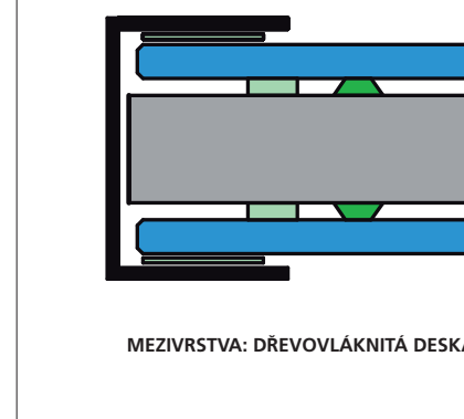
KONSTRUKCE DVEŘÍ
