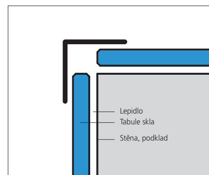
ROHOVÝ PROFIL: ÚHELNÍK
