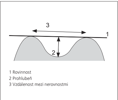
MĚŘENÍ ROVINNOSTI
