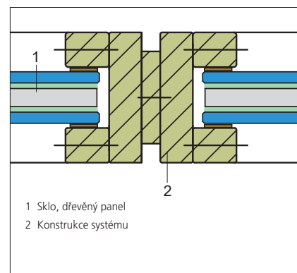
DŘEVĚNÁ KONSTRUKCE: VODOROVNÝ PRŮŘEZ
