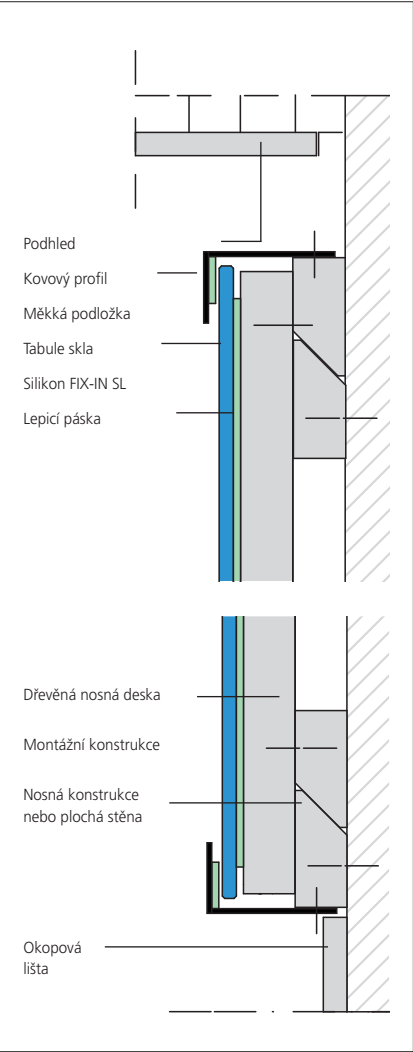
SVISLÝ ŘEZ
