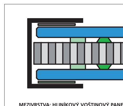
MEZIVRSTVA: HLINÍKOVÝ VOŠTINOVÝ PANEL
