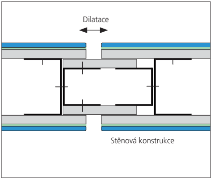
DILATAČNÍ SPÁRA: ZEĎ
