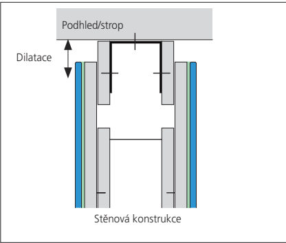
POSUVNÁ SPÁRA: PODHLED/STROP
