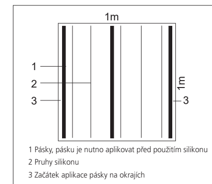
APLIKACE LEPIDEL
