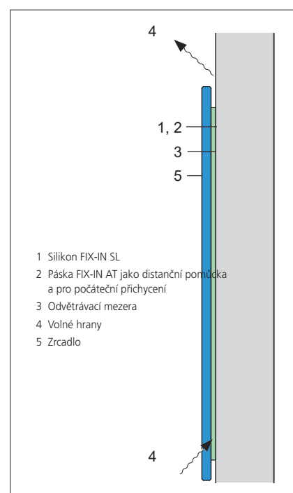
SVISLÝ ŘEZ
