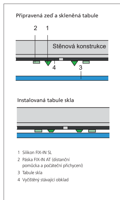
SKLO BEZ BEZPEČNOSTNÍ FÓLIE
