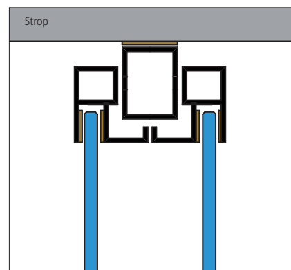
KOVOVÁ KONSTRUKCE: SVISLÝ PRŮŘEZ
