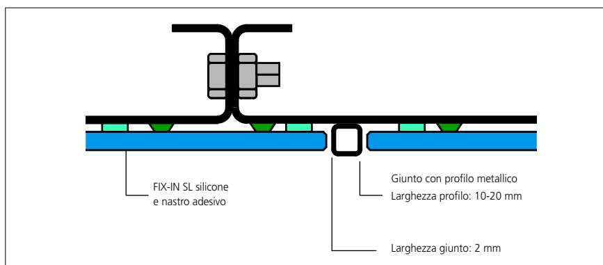
CABINA ASCENSORE: SEZIONE TRASVERSALE ORIZZONTALE CON GIUNTO PROFILATO
