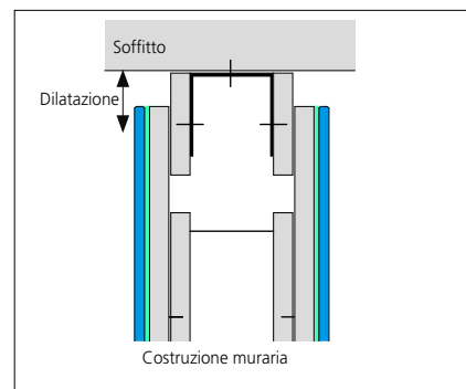
GIUNTO SCORREVOLE SOFFITTO
