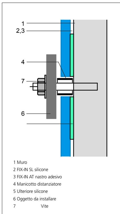
INSTALLAZIONE CON MANICOTTI
