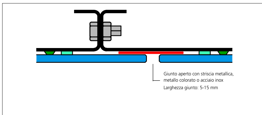
CABINA ASCENSORE: SEZIONE TRASVERSALE ORIZZONTALE CON GIUNTO COLORATO
