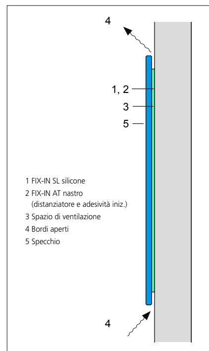
SEZIONE VERTICALE
