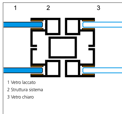
STRUTTURA METALLICA: SEZIONE TRASVERSALE ORIZZONTALE
