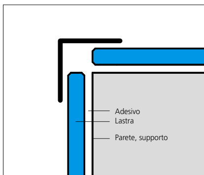
PROFILI ANGOLARI: PROFILO ANGOLARE
