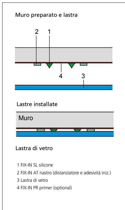
VETRO SENZA PELLICOLA DI SICUREZZA
