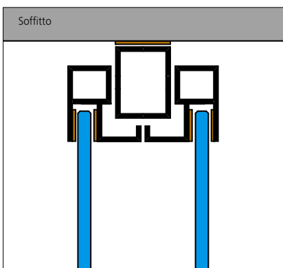
STRUTTURA METALLICA: SEZIONE TRASVERSALE VERTICALE
