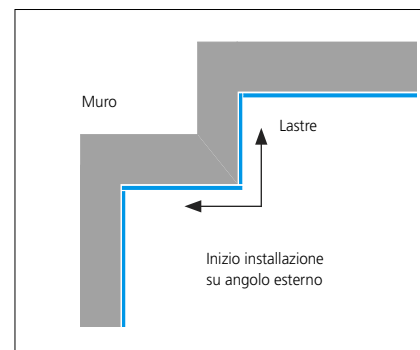
MONTAGGIO: PIANTA PAVIMENTO
