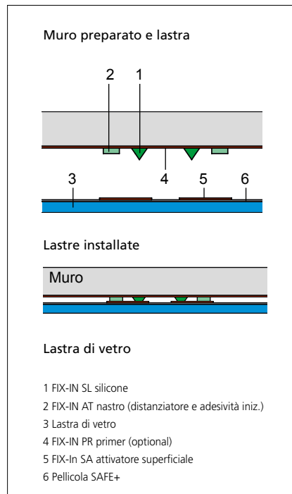
VETRO CON PELLICOLA SAFE+
