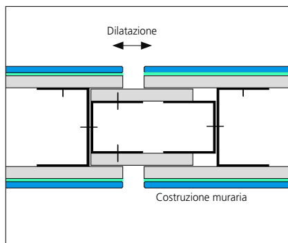
GIUNTO DI DILATAZIONE: MURO
