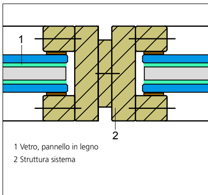
COSTRUZIONE IN LEGNO: SEZIONE TRASVERSALE ORIZZONTALE
