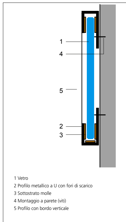
MONTAGGIO MECCANICO: MIROX
