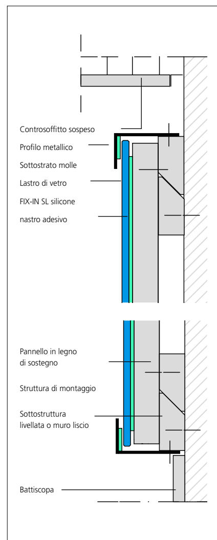
SEZIONE TRASVERSALE VERTICALE
