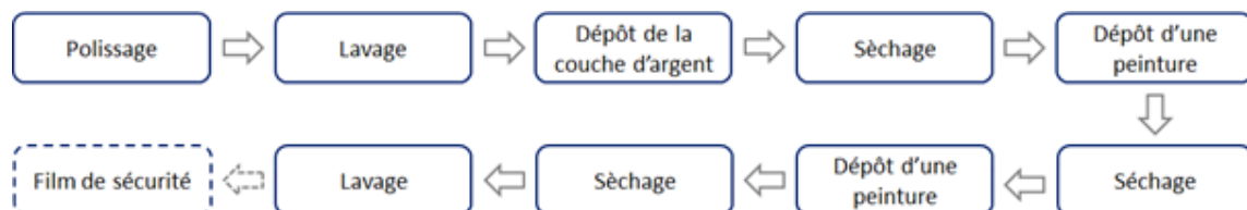
Figure 3 : Etapes de production d'un miroir Mirox MNGE
